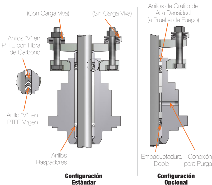
EMPAQUETADURA PT (FIGURA 13)
