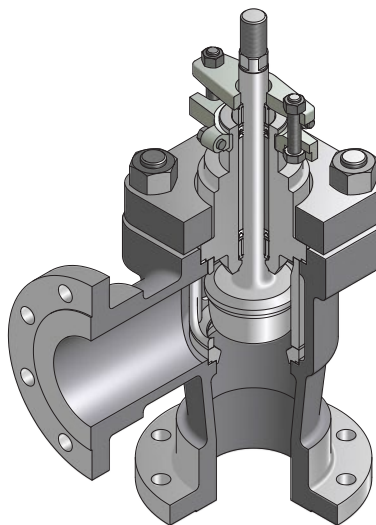
CUERPO ESTILO ANGULAR (FIGURA 2)
