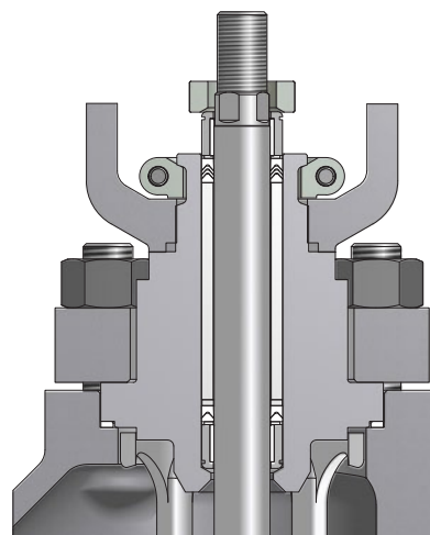
BRIDA DE TAPA (FIGURA 8)
