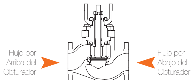
SENTIDO DE FLUJO (FIGURA 20)
