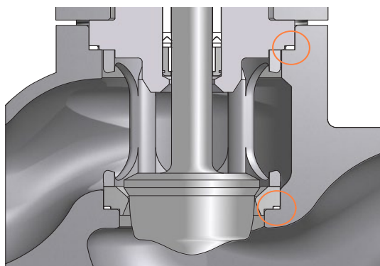
JUNTAS DEL CUERPO (FIGURA 9)
