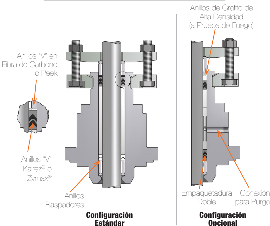
EMPAQUETADURA PTG & PTG-XT (FIGURA 14)
