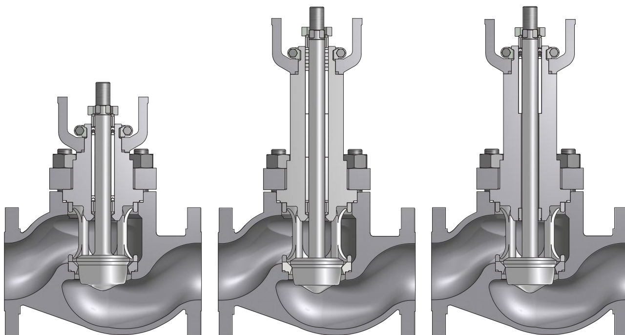
TIPOS DE TAPAS PARA GLS (FIGURA 11)
